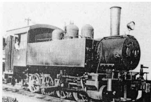
蒸気機関車 1号機アメリカ製
